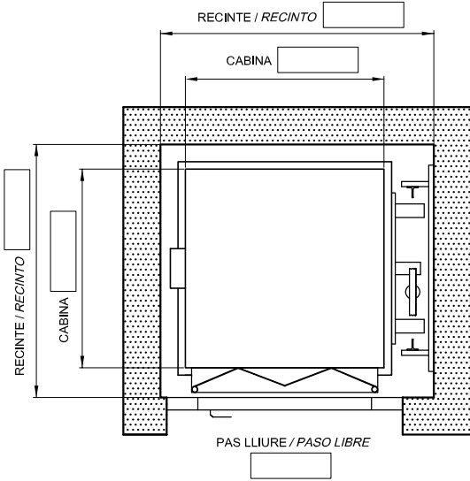
SIMPLE EMBARQUE TRASERO
